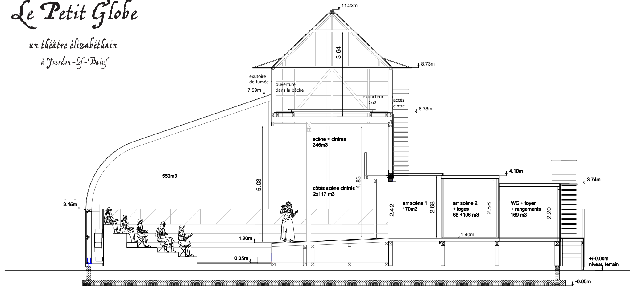
Coupe A-A
